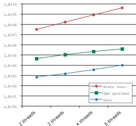
FIG. 8 – Évolution de l'espace d'états concret et du graphe quotient dans la modélisation du \mu Broker.
